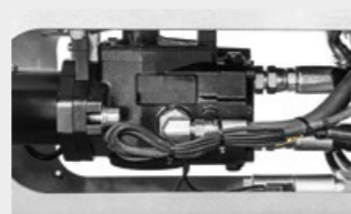
Moteur hydraulique à pistons à débit variable de 17 à 34 cc avec soupape de sécurité et fonction anticavitation intégrée
